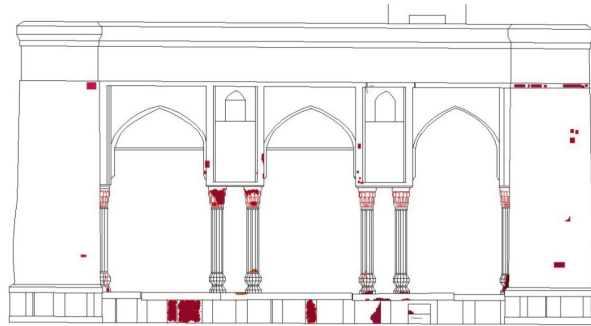
شکل ۳- آسیب‌های بنای خدایخانه در صحن مسجد جامع عتیق شیراز (لگه‌ها بیانگر آسیب‌هاست)
